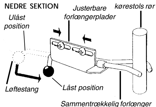
FIGUR 2 - INSTALLERING AF ULTI-MATE LUFTRYGLÆN TIL NEDRE RYGLÆNS RØR
